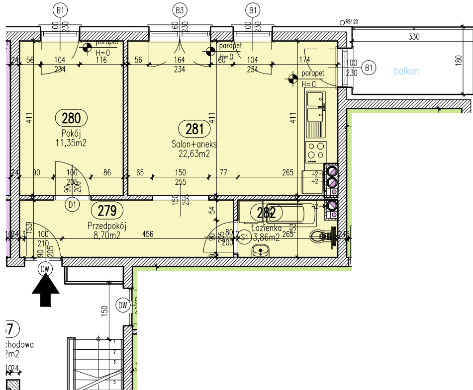
RZUT MIESZKANIA G-44 SKALA 1:100
