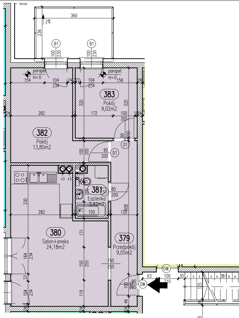
RZUT MIESZKANIA F-48 SKALA 1:100
