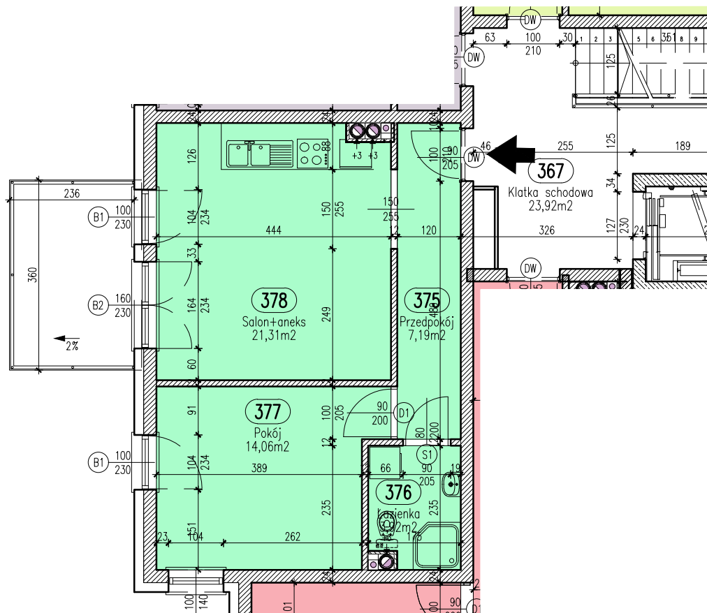
RZUT MIESZKANIA F-47 SKALA 1:100
