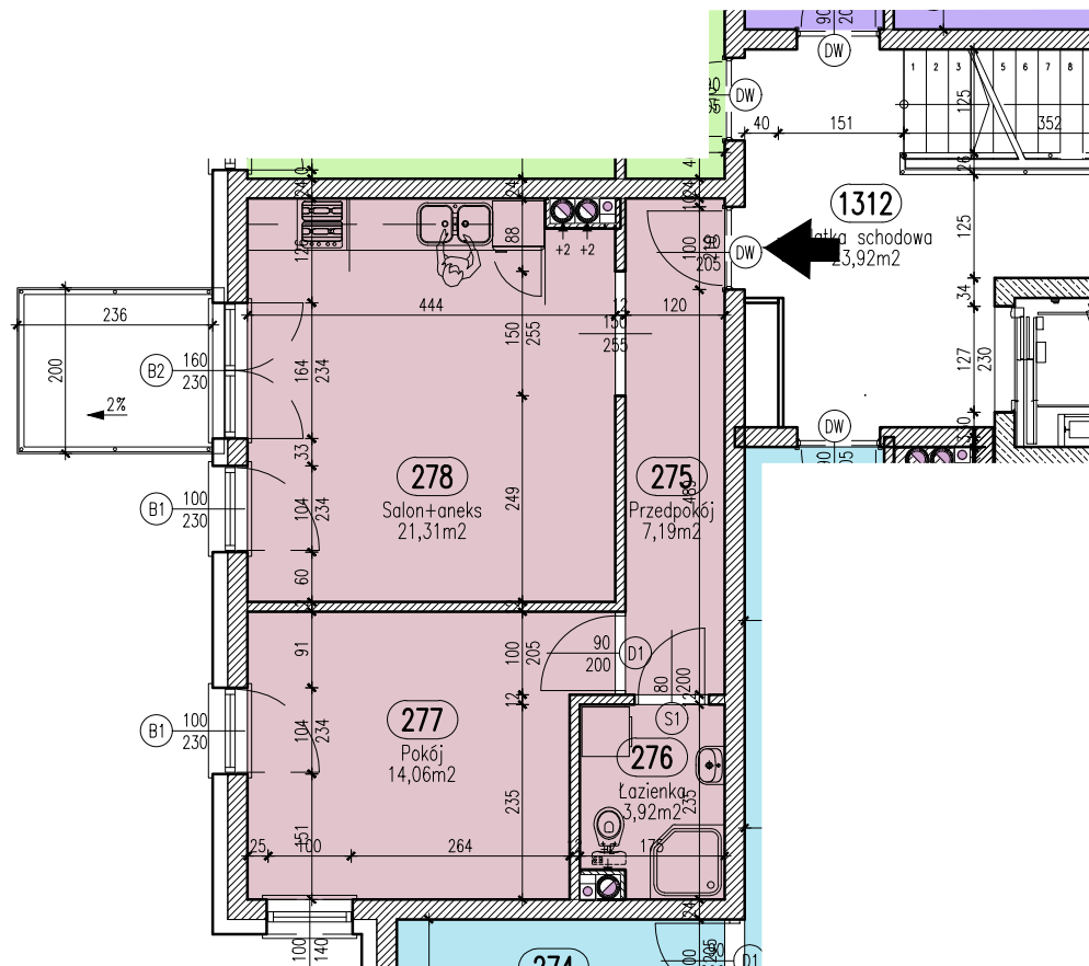
RZUT MIESZKANIA F-43 SKALA 1:100
