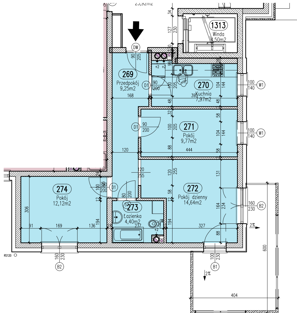
RZUT MIESZKANIA F-42 SKALA 1:100
