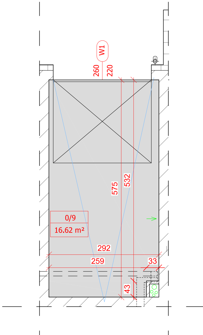
Rzut garażu skala 1:50
